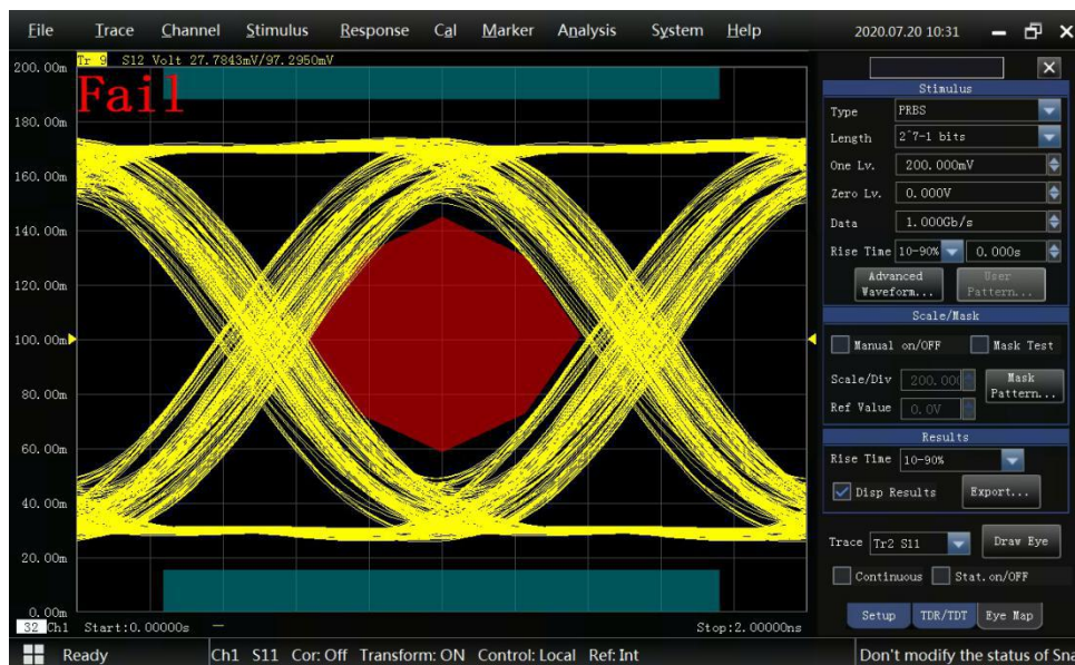
Add Jitter
