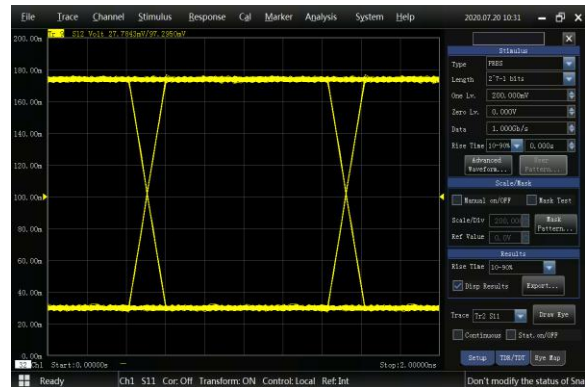
Add Noise
