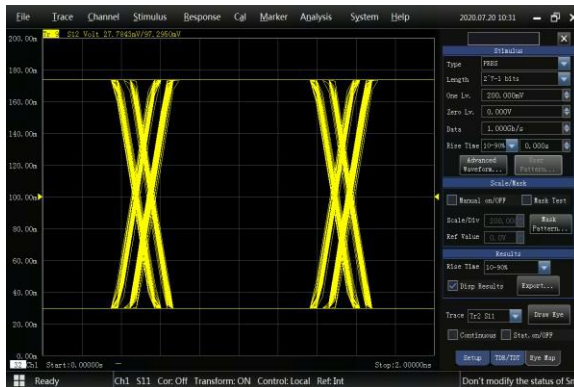
Add Jitter
